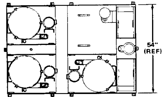
RCS 90
