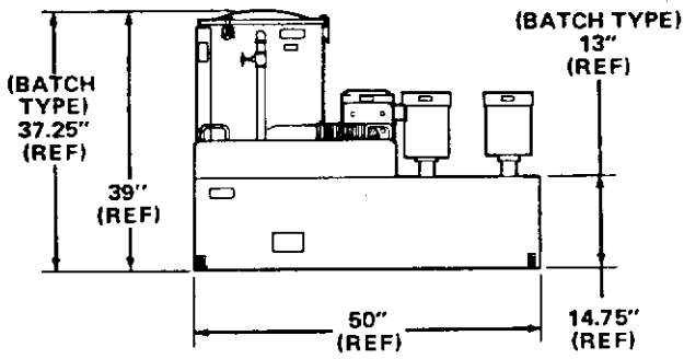
RCS 30
