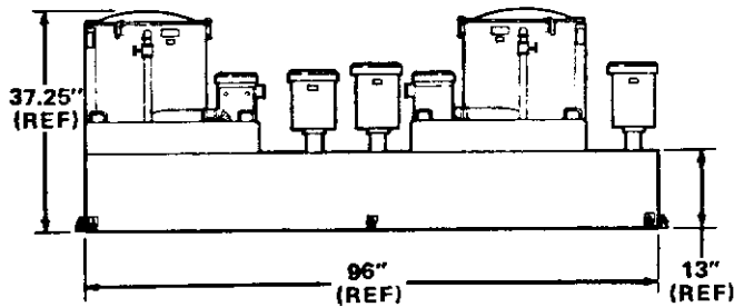
RCS 120
