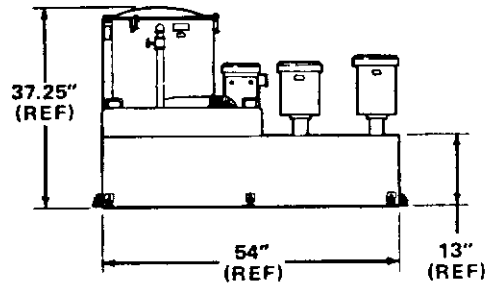
RCS 60
