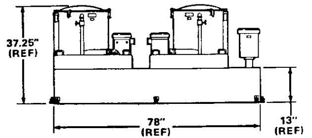
RCS 90
